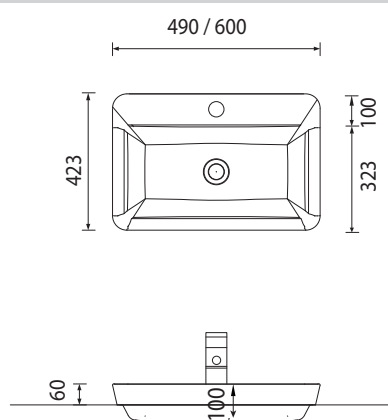
Mineralguss - Aufsatzwaschtisch WTA S111 / WTA S112 eingelassener Waschtisch
