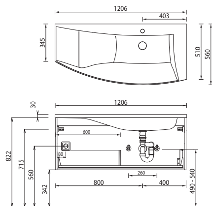
SWM 112L
