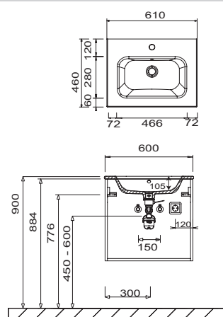
WTM54061 Unterschrankhöhe 560 mm
