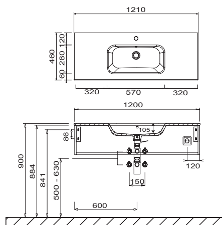
WTM54121 Unterschrankhöhe 280 mm
