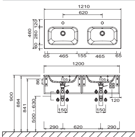
WTM542D1 Unterschrankhöhe 280 mm
