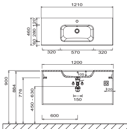
WTM54121 Unterschrankhöhe 560 mm
