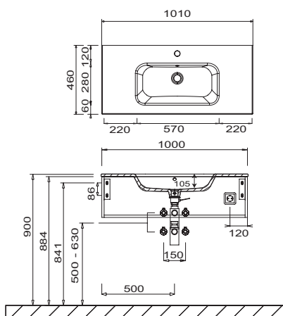
WTM54101 Unterschrankhöhe 280 mm
