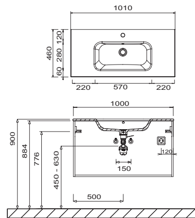
WTM54101 Unterschrankhöhe 560 mm
