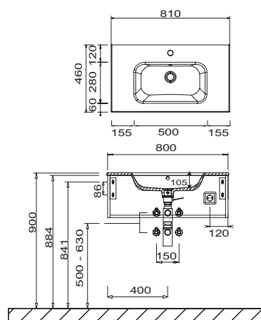
WTM54081 Unterschrankhöhe 280 mm
