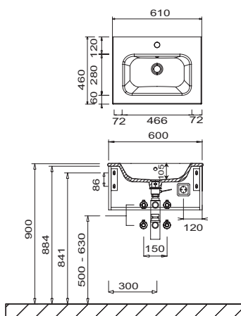
WTM54061 Unterschrankhöhe 280 mm
