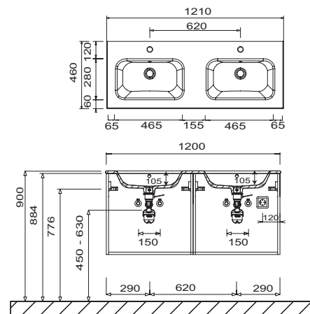
WTM542D1 Unterschrankhöhe 560 mm
