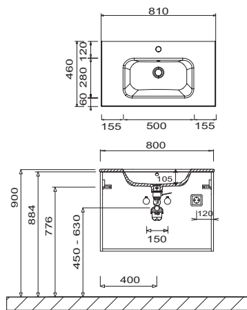
WTM54081 Unterschrankhöhe 280 mm
